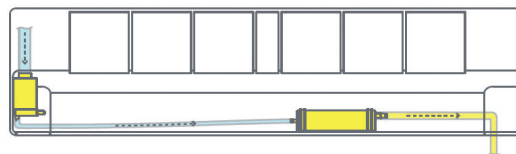
Watersensor verticaal en pomp horizontaal in het binnentoestel.
