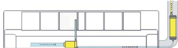
Watersensor in het binnentoestel, pomp buiten het toestel.
